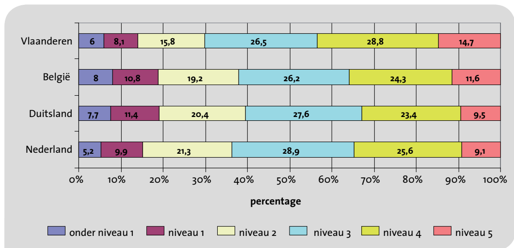
Figuur 9.4.2 Percentage leerlingen per vaardigheidsniveau op de leesvaardigheidsschaal
