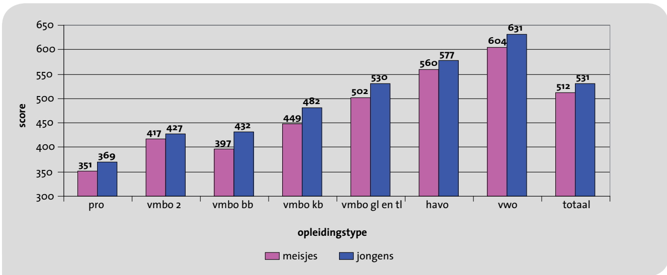
Figuur 2.3.13 Gemiddelde scores van meisjes en jongens in Nederland op de vaardigheidsschaal natuurwetenschappen: competentie Gebruikmaken van bewijzen
