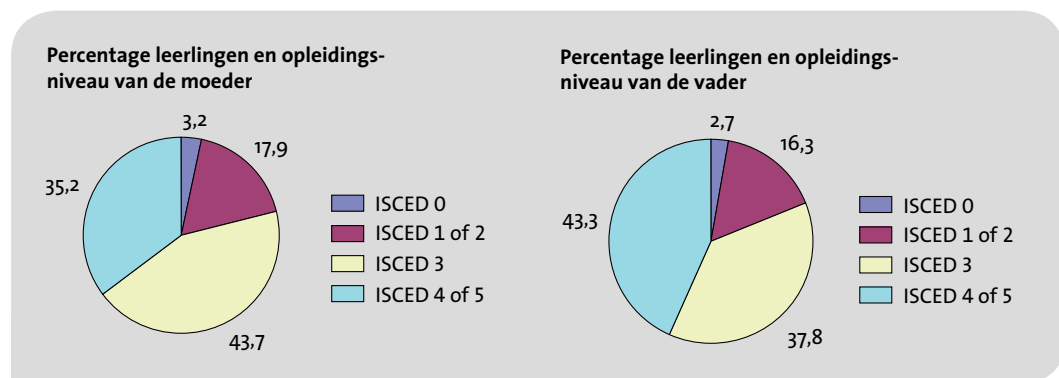
Figuur 7.4.2a en 2b Percentage leerlingen dat een moeder resp. vader heeft met een opleidingsniveau op de ISCED schaal van 0 – 5
